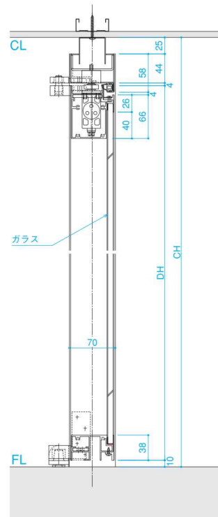
■B-B断面
