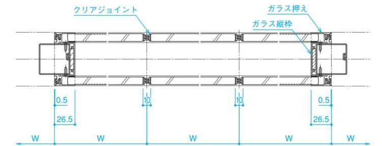
■E-E断面
