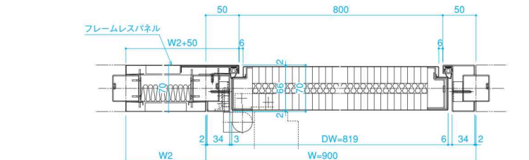
■D-D断面
