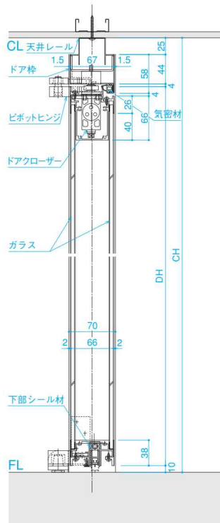
■D-D断面
