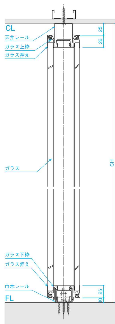
■B-B断面
