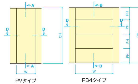
■立面図
