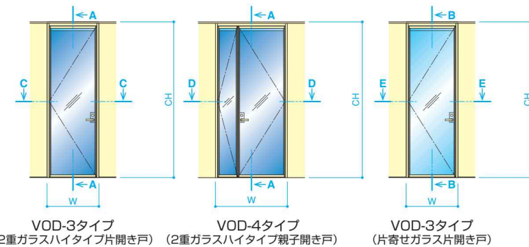
■立面図
