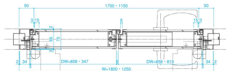
■E-E断面
