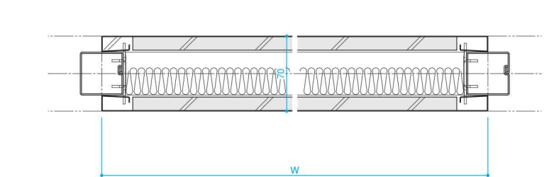
■D-D断面
