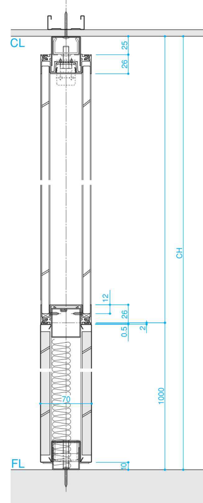
■D-D断面
