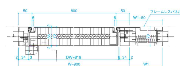
■B-B断面
