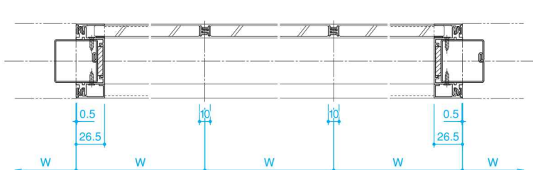
■G-G断面
