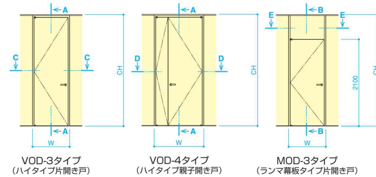
■立面图
