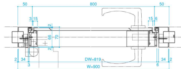
■E-E断面
