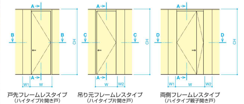
■立面図
