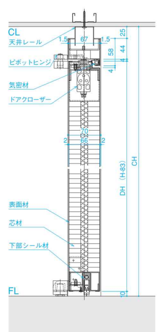
■A-A断面
