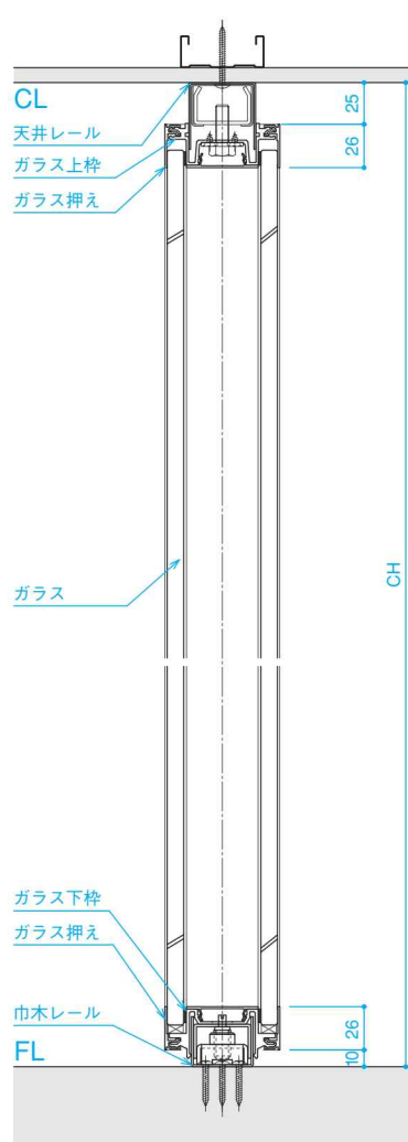
■A-A断面
