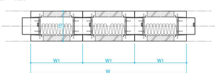
■H-H断面
