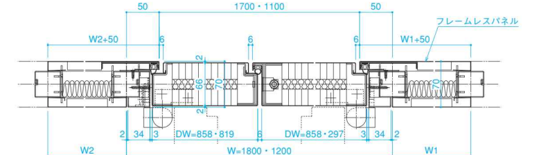
■D-D断面
