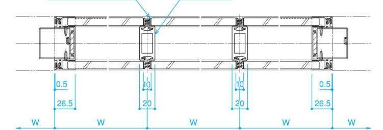
■F-F断面
