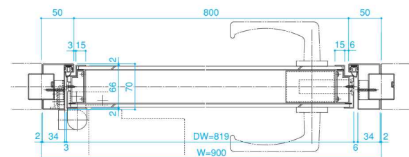
■C-C断面
