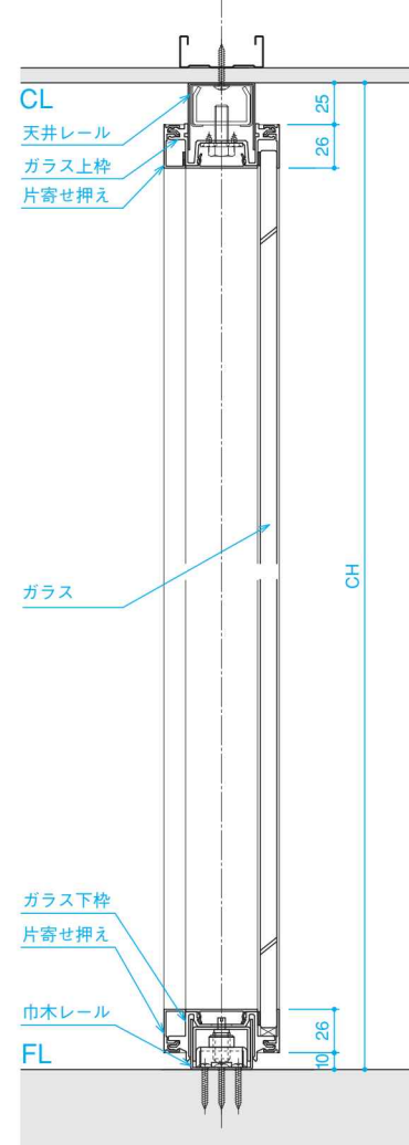
■C-C断面
