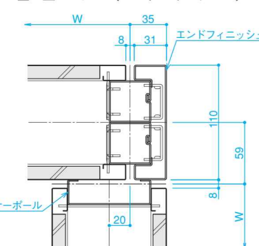
■L型コーナー（エンドフィニッシュ）
