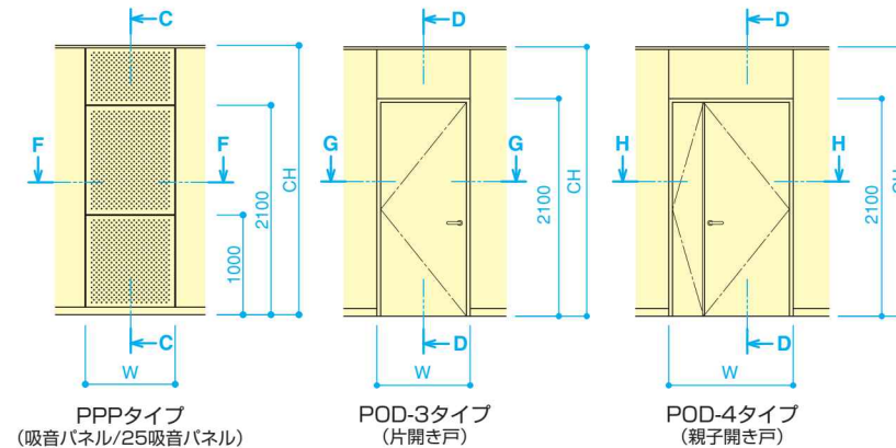
■製品寸法
