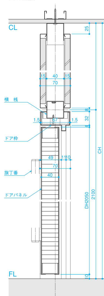
■D-D断面
