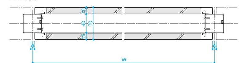
■F-F断面
