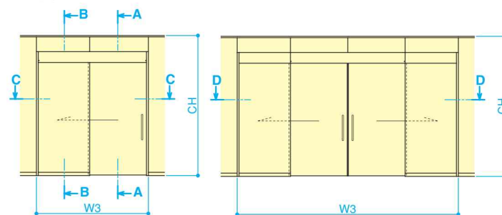
カームドア内蔵タイプ (片引き)
