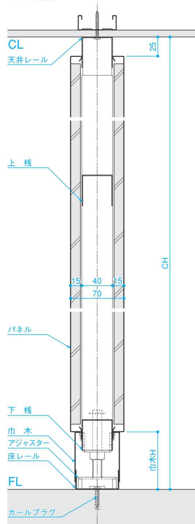
■A-A断面
