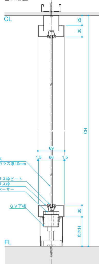
■C-C断面
