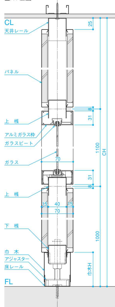
■A-A断面
