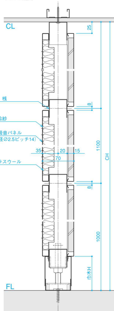
■C-C断面
