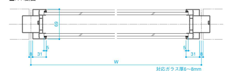
■H-H断面
