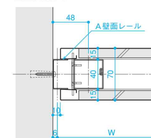
■壁面納まりA
