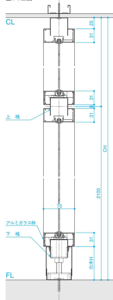
■B-B断面
