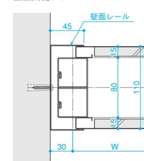
■壁面納まりB
