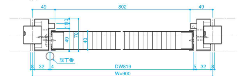
■H-H断面
