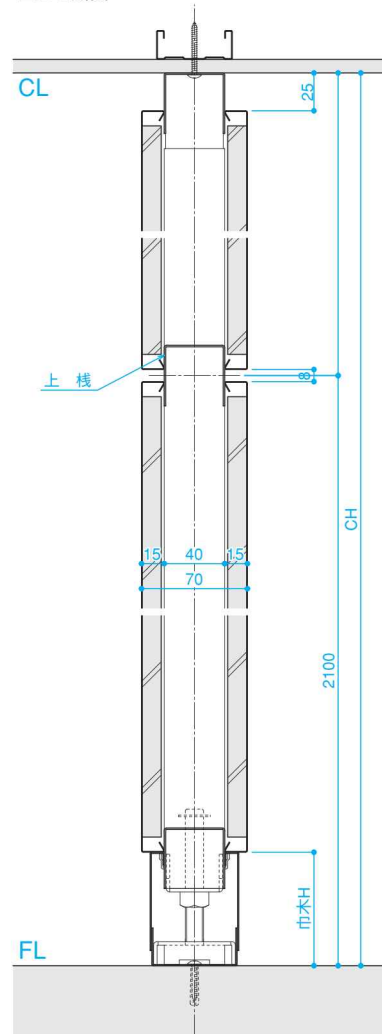
■B-B断面
