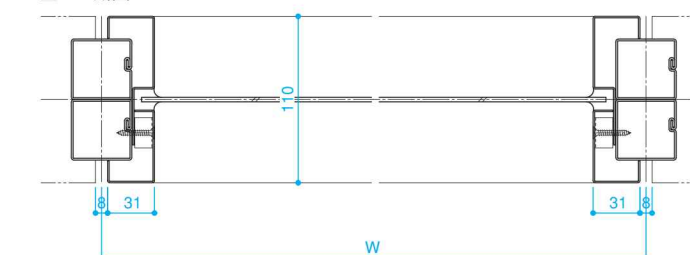
■C-C断面
