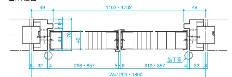
■H-H断面
