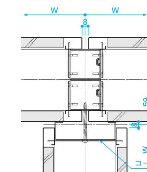
■T型コーナー詳細
