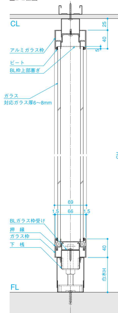
■D-D断面
