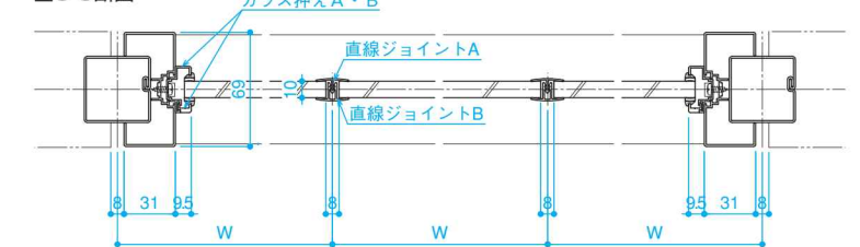
■G-G断面
