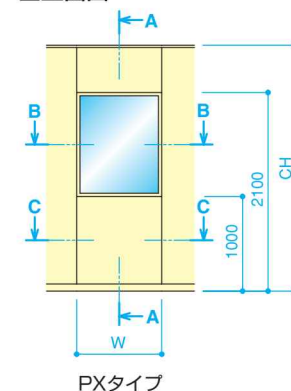
■立面図
