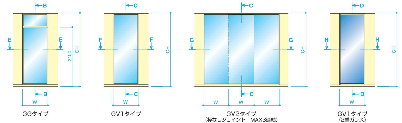
■製品寸法（全面ガラス）
