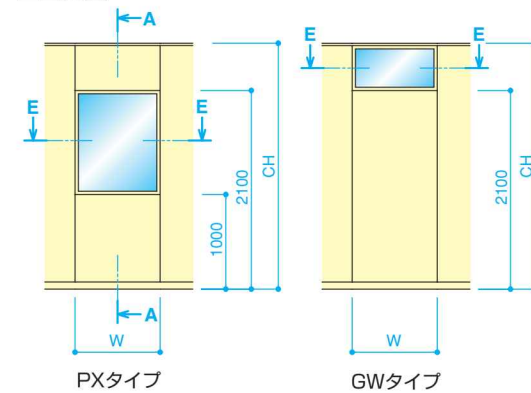
■立面図
