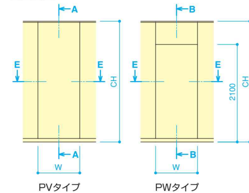
■立面図
