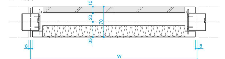
■G-G断面
