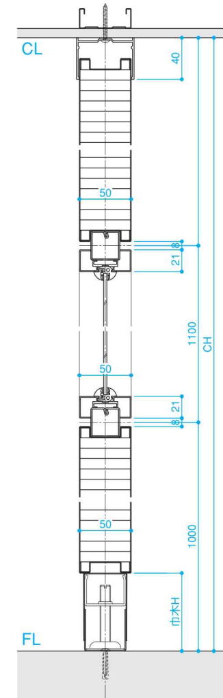
■C-C断面
