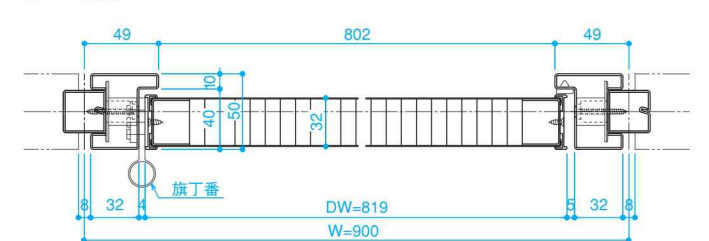
■H-H断面
