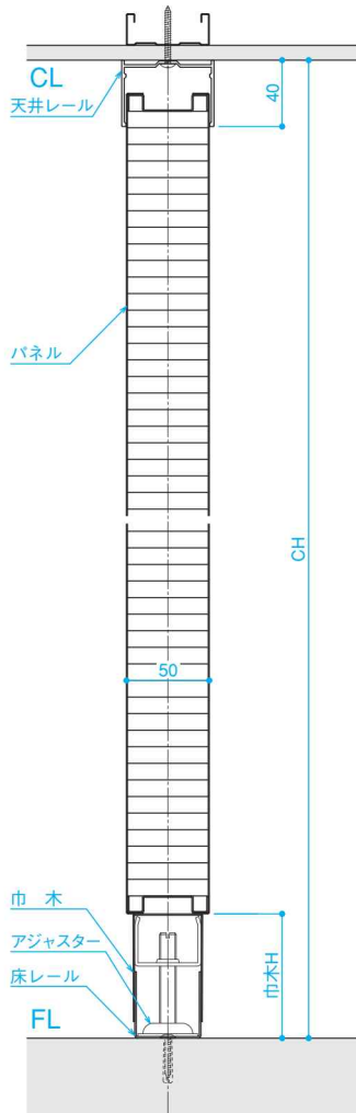
■A-A断面
