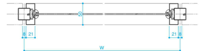
■G-G断面
