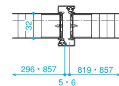
■I-I断面
