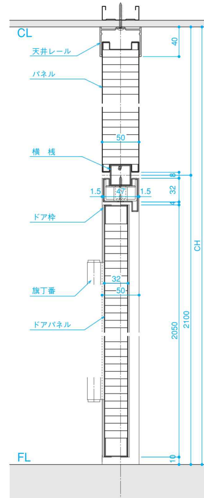
■D-D断面
