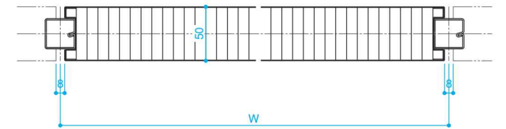
■F-F断面
