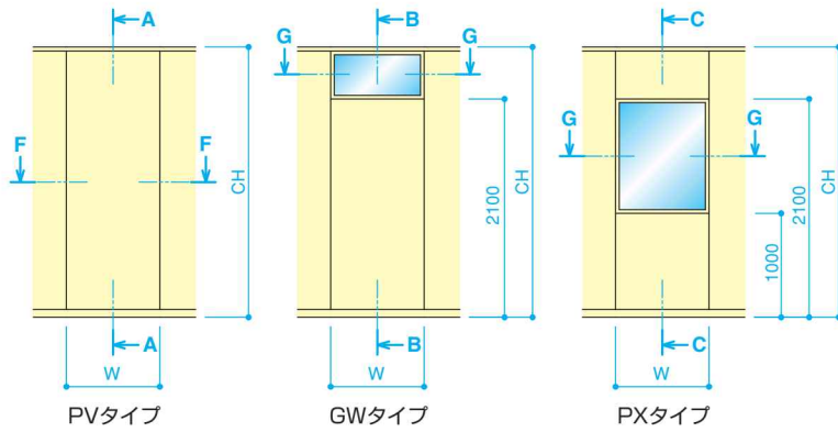
■立面図
