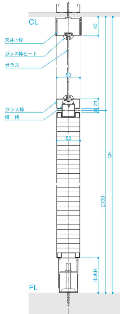
■B-B断面
