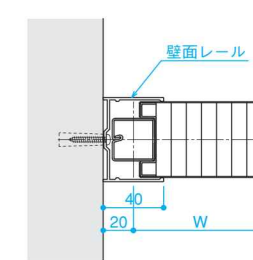
■壁面納まり
